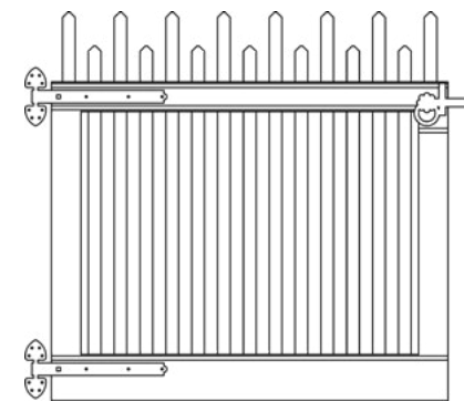
Style G2
