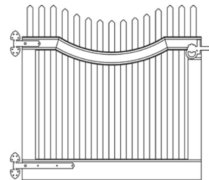
Style G3
